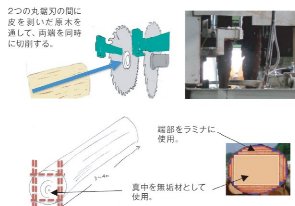
図2 導入したツイン丸鋸
