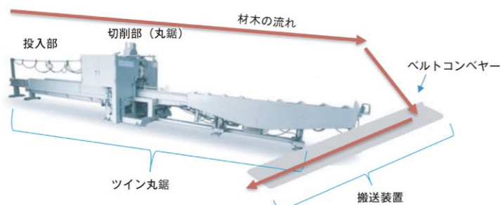
図1 ツイン丸鋸構成図
